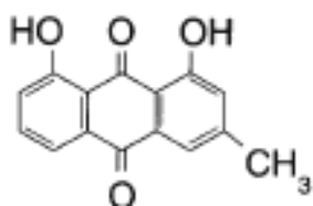
Chrysofanol
