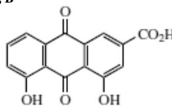
Rhein
