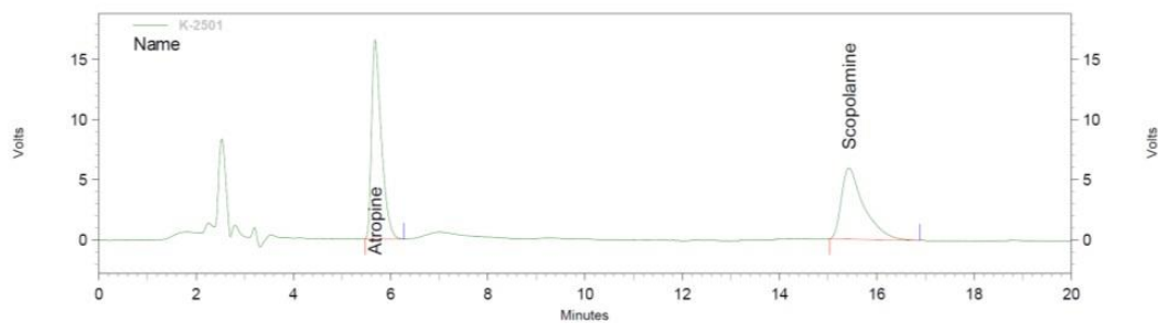
شکل شماره ۱- نمونه کروماتوگرام HPLC آتروپین و اسکوپولامین اندام گیاهی (الف) و محلول استاندارد (ب)
