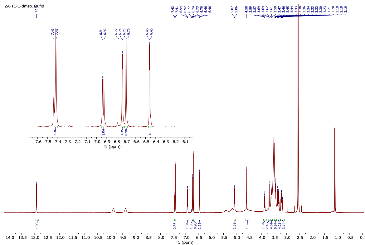
شکل ۲. طیف H NMR ترکیب شماره ۱، Luteolin 7-O-rutinoside (طیف سنج ۵۰۰ مگا هرتز، حلال DMSO دو تریه)
