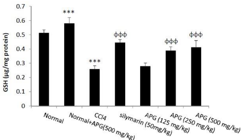
شکل ۴. میزان تغییرات گلو تاتیون احیاء در گروه‌های مختلف. *** نشانگر تفاوت معنی‌دار در مقایسه با گروه نرمال ( P < 0/001 ) و **** نشانگر تفاوت معنی‌دار در مقایسه با گروه سمی ( P < 0/001 ) می‌باشند. نتایج به صورت انحراف معیار \pm میانگین بیان شده است. عصاره آبی گلنار (APG) و گلو تاتیون احیاء (GSH).
