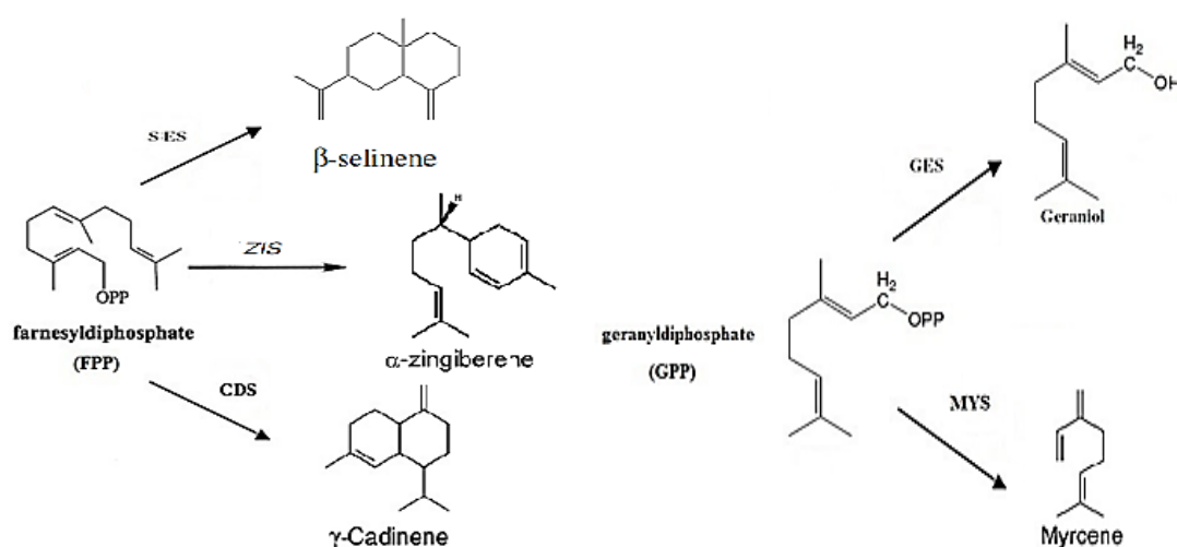
شکل ۱. نحوه بیوسنتز بتا-میرسین، ژرانیول و گاما-کادینن در ریحان، (SES) Selinene synthase، (MES) beta-myrcene synthase، (ZIS) alpha-zingiberene synthase و (GES) Geraniol synthase و (CDS) cadinene synthase
