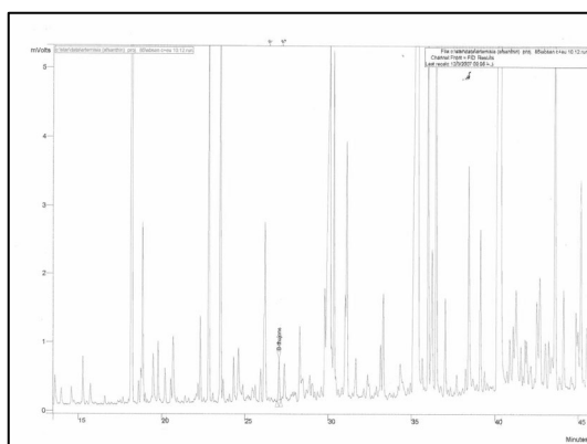
شکل شماره ۲- کروماتوگرام GC اسانس گل های گیاه افسنطین
