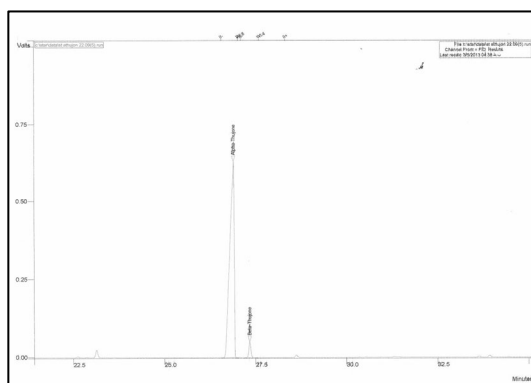
شکل شماره ۱- کروماتوگرام GC مخلوط استانداردهای \alpha و \beta توجون
