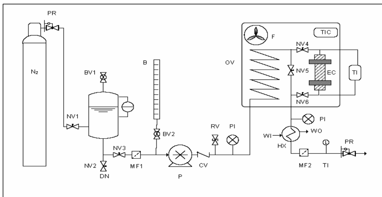
شکل شماره ۲- دیاگرام سیستم استخراج با آب فوق گرم
