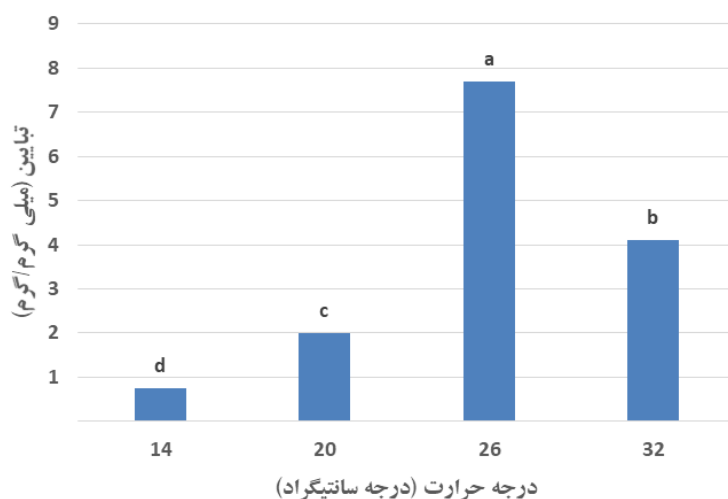
شکل شماره ۴- مقایسه میانگین اثر دما بر تباین ریشه‌های نابجا خشک‌شده کبیر ( P \leq 0.05 )
