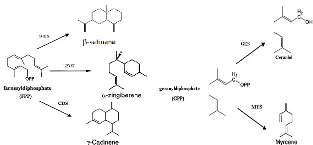
شکل ۱. نحوه بیوسنتز بتا-میرسین، ژرانیول و گاما-کادینن در ریحان، (SES) Selinene synthase، (MES) beta-myrcene synthase، (MES) gamma-geraniol synthase و (ZIS) alpha-zingiberene synthase و (GES) Geraniol synthase و (CDS) cadinene synthase
