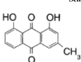
Chrysofanol
