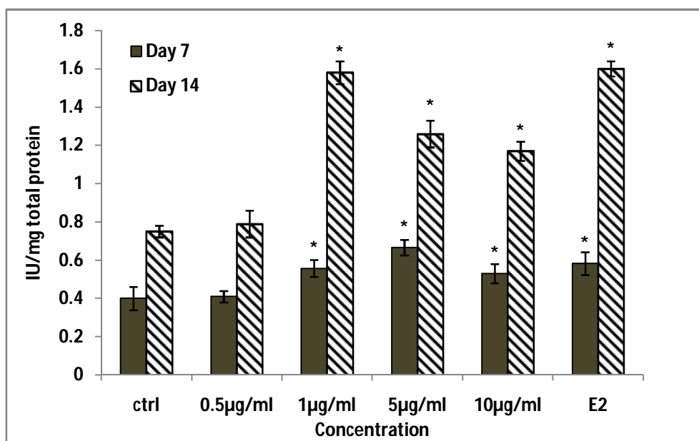
نمودار شماره 3- الگوی تأثیر عصاره ریشه گیاه باریجه و تیمار 17- بتا استرادیول (E2) بر میزان فعالیت آنزیم آلکالین فسفاتاز در بازه‌های زمانی 7 و 14 روز پس از القاء تمایز، * نشان‌دهنده‌ی معنی‌داری نتایج در مقایسه با گروه کنترل می‌باشد (p ≤ 0/5)
