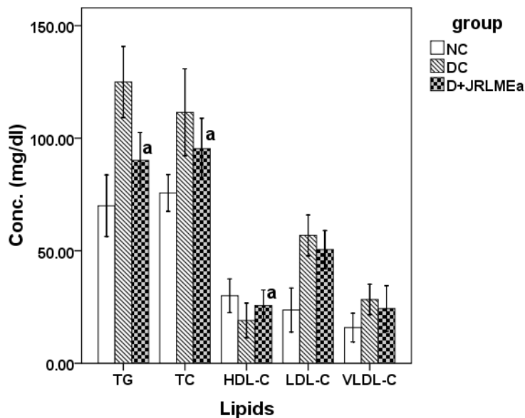
نمودار شماره ۴- اثر JRLMEa بر میزان لیپیدهای خون. NC: گروه شاهد سالم، DC: گروه شاهد دیابتی، D+JRLMEa: گروه دیابتی دریافت کننده عصاره JRLME در دوز ۲۵۰ mg/kg. p < 0.001 ; a : در مقایسه با گروه DC.
