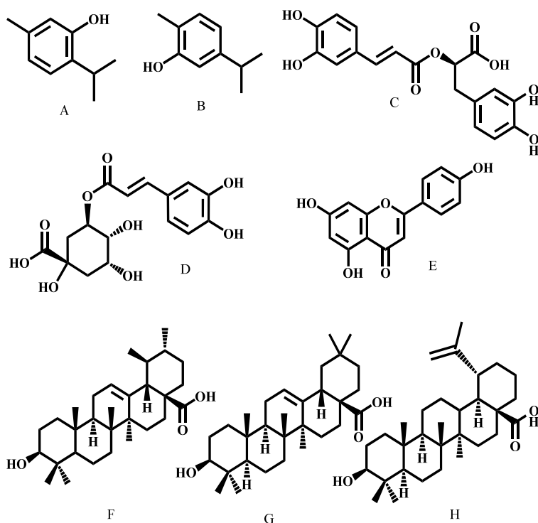
شکل شماره ۱- ساختار شیمیایی معروف‌ترین متابولیت‌های ثانویه موجود در گونه‌های مختلف آویشن، (A تیمول، B کارواکرول، C رزمارینیک اسید، D کلروزنیک اسید، E آپیجین، F اورسولیک اسید، G اولئانولیک اسید، H بتولینیک اسید)
