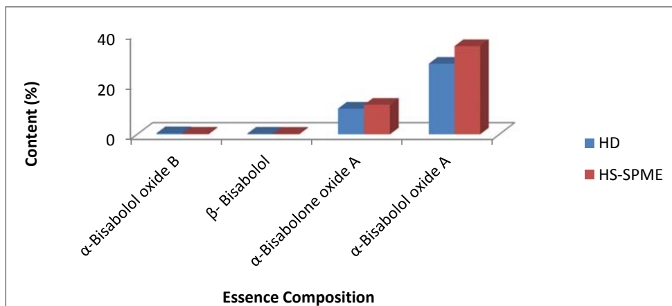
شکل شماره ۲- مقایسه الف- مونوترپن‌های هیدروکربنی ب- مونوترپن‌های اکسیژن‌دار ج- سزکوئی‌ترین‌های اکسیژن‌دار شناسایی شده اسانس گیاه F. imperialis به روش‌های HD و HS-SPME
