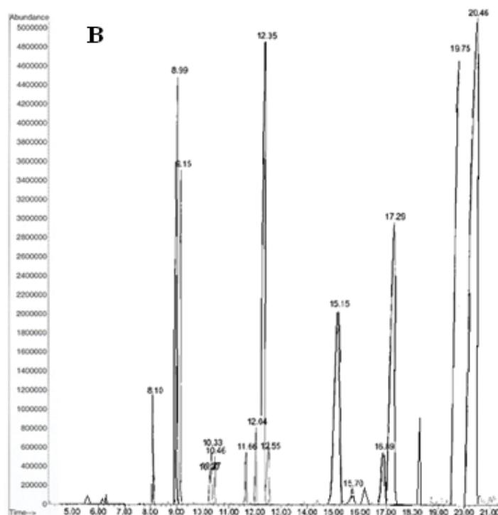
شکل شماره ۱- کروماتوگرام گازی ترکیبات روغن اسانسی گیاه Fritillaria officinalis به روش HS-SPME (B) HD (A)
