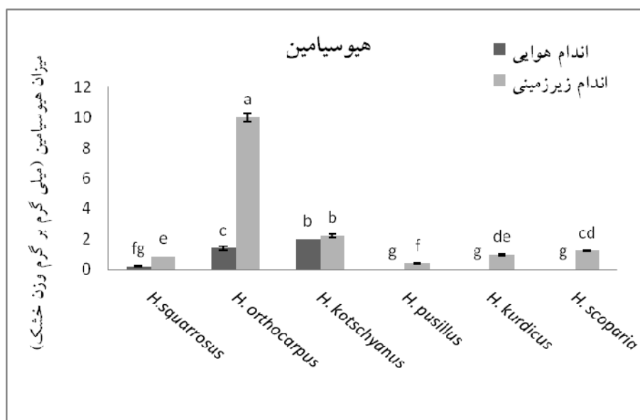
نمودار شماره ۱- میزان هیوسیامین در اندام‌های هوایی و زیرزمینی گونه‌های مختلف جنس Hyoscyamus spp. ستون‌های دارای حداقل یک حرف مشترک، اختلاف معنی‌داری در سطح احتمال ۵ درصد با یکدیگر ندارند.
