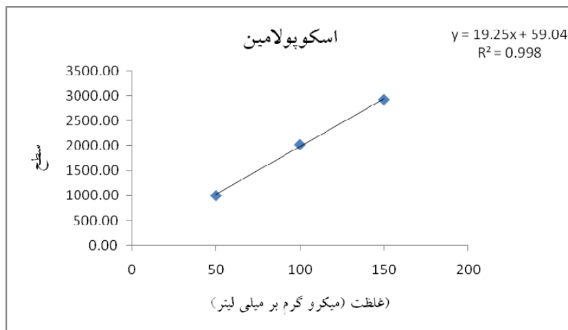
منحنی شماره ۲- منحنی کالیبراسیون ترکیب اسکوپولامین
